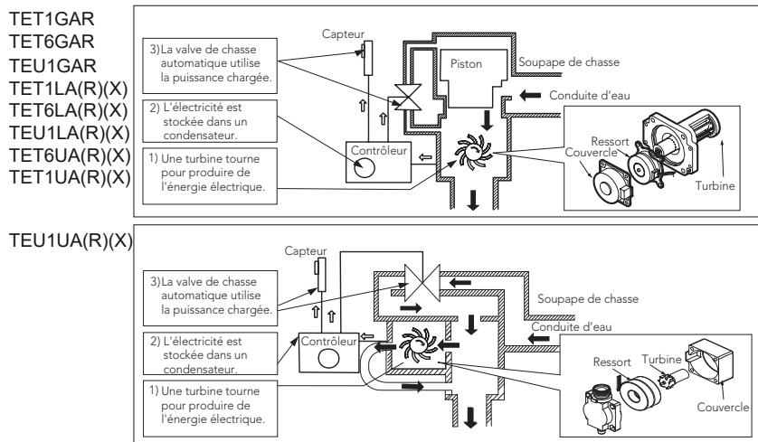
fig. 1 Générateur Hydropowered
