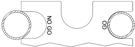
Figura 3 – Una buena conexión
