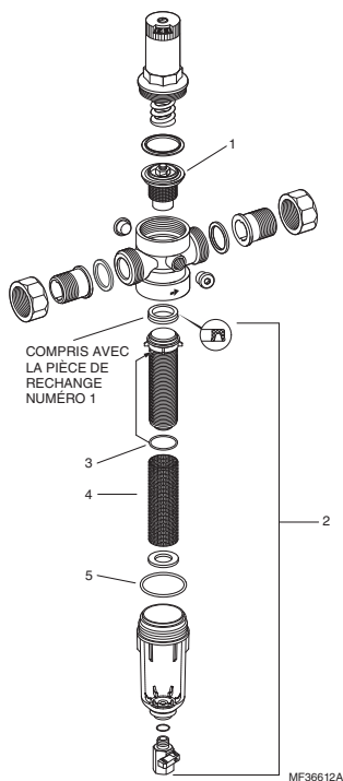
Fig. 5. Schéma des pièces de rechange.
