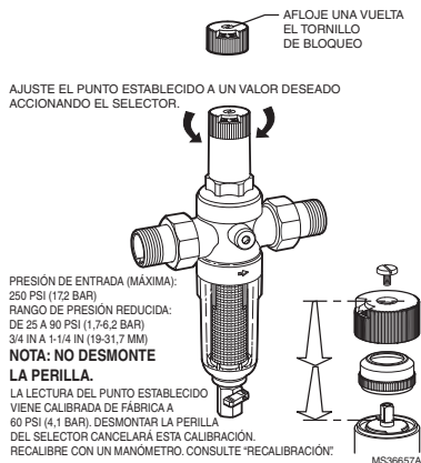
Fig. 2. Cambiar presión de salida.
