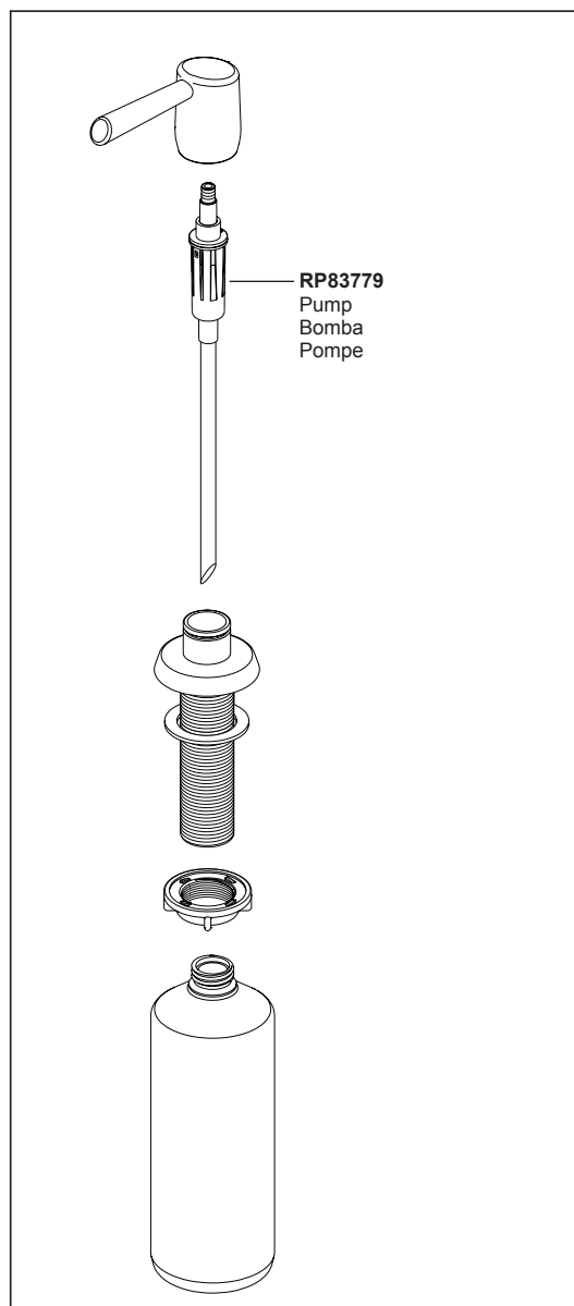
RP100736▲ Dispenser Assembly Ensamble del Dispensador Distributeur
