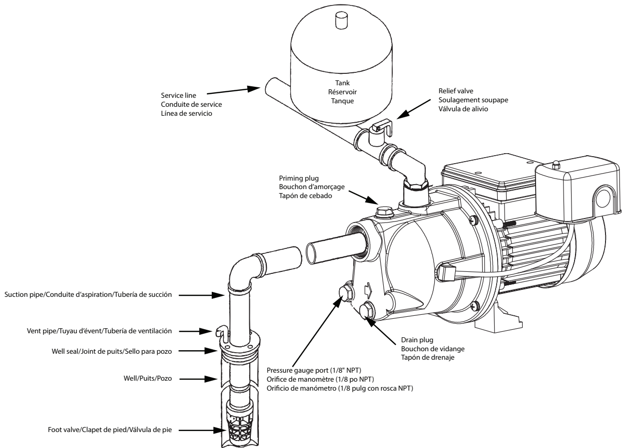
FIGURE 5 • FIGURE 5 • FIGURA 5 SHALLOW WELL - INLINE TANK (WITH FOOT VALVE) • PUIITS PEU PROFOND, RÉSERVOIR EN LIGNE (AVEC CLAPET DE PIED) • POZO POCO PROFUNDO, TANQUE EN LÍNEA (CON VÁLVULA DE ASPIRACIÓN)
