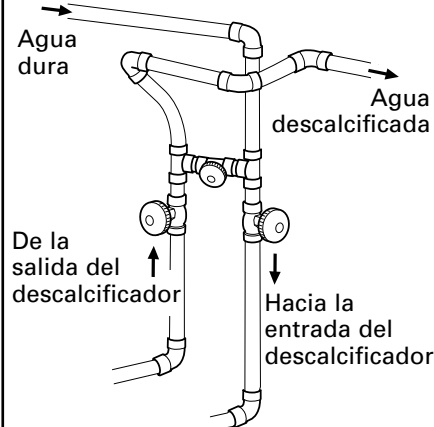
Fig. 2 VÍA DE ENLACE Úsela si el flujo de suministro fluye desde la izquierda. Incluya una derivación sencilla o de 3 válvulas.
