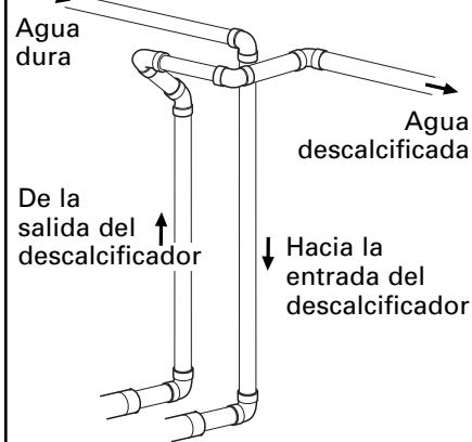
Fig. 1 VÍA DE ENLACE Úsela si el flujo de suministro fluye desde la izquierda. Incluya una derivación sencilla o de 3 válvulas.
