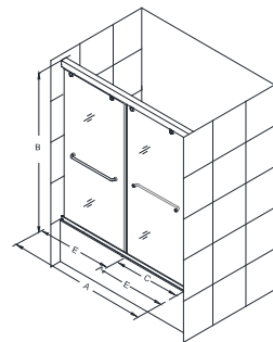
Configuration 2 (Tub)
